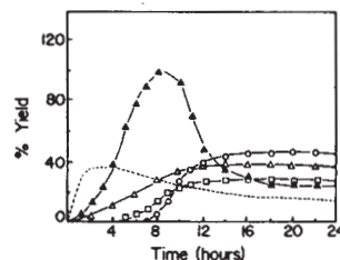
Figure 2. Product formation vs. time for CAN-C 6 H 5 CH 3 -CH 3 NO 2 : \Delta , CH 3 C 6 H 4 CH 2 NO 2 ; \circ , CH 3 C 6 H 4 CHO; \square , C 6 H 5 CHO, \nabla , CH 3 C 6 H 4 NO 2 ; --, C 6 H 5 CH 2 OAc.
